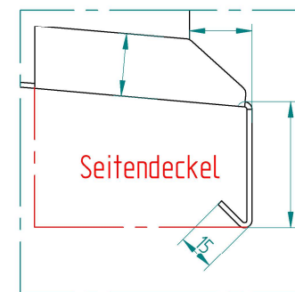
EINZELHEIT A
