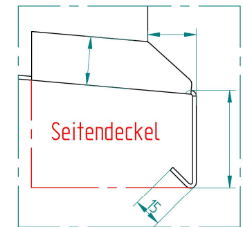
EINZELHEIT A
